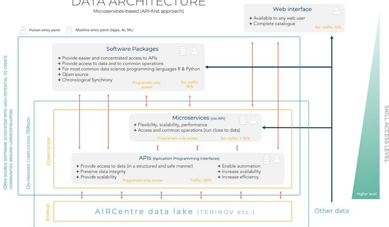
Figura 28 – Concepção e arquitectura do sistema para a gestão dos dados no centro de dados do AIR Data
